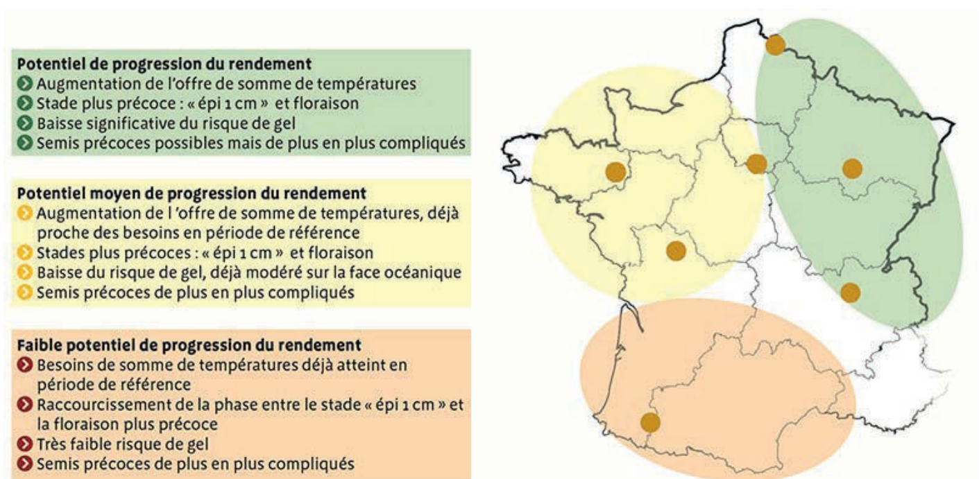
Figure 8. Impact de la hausse des températures sur le rendement des CIVE d'hiver d'une région à l'autre
